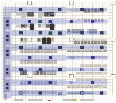
图 6 优化后的风口布置图
