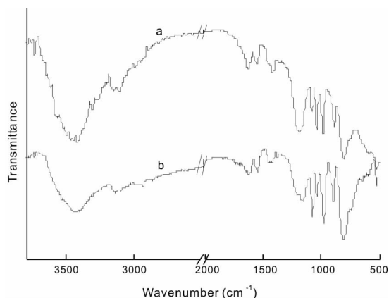
图 8 新鲜催化剂 (a) 和使用 5 次后催化剂 (b) 的红外谱图
