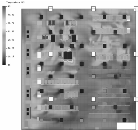
图 7 优化后机房温度场模拟
