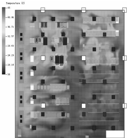
图 4 机房温度场模拟结果
