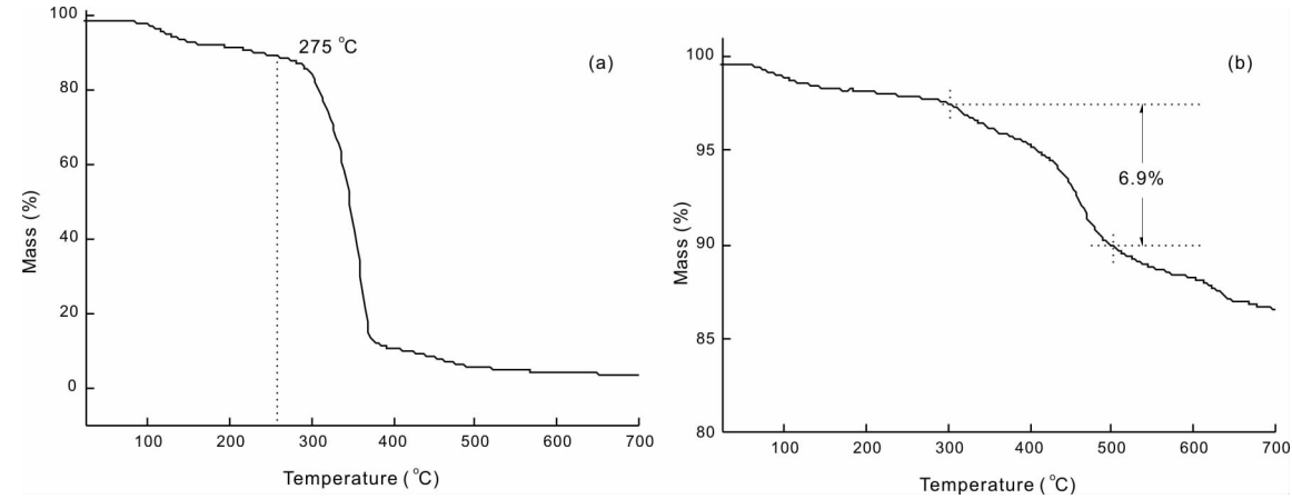
图 6 Poly( VMPS) (a) 与 Poly( VMPS) – H 2 PW (b) 的 TG 谱图
