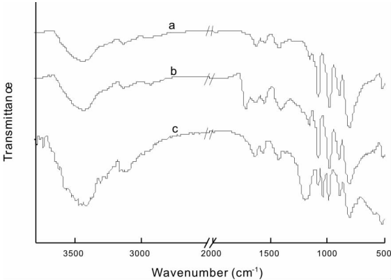
图5 聚合类杂多化合物的红外谱图 (a) Poly(VPIM)-H 2 PW; (b) Poly(VMCA)-H 2 PW; (c) Poly(VMPS)-H 2 PW
