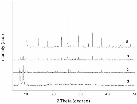
图2 不同试样的XRD谱图 (a) Pure H3PW12O40; (b) VMPS-H 2 PW (c) VMCA-H 2 PW; (d) VPIM-H 2 PW
