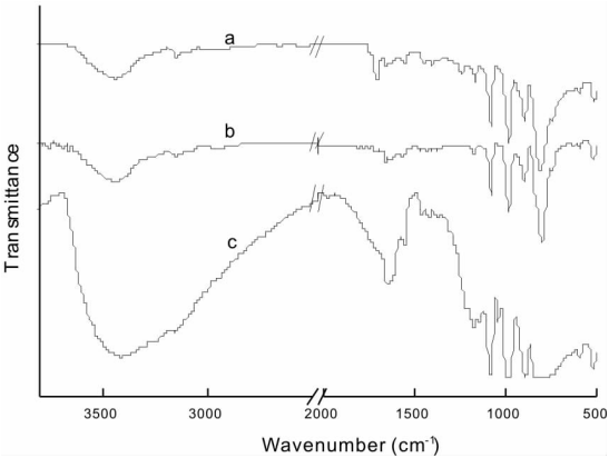
图4 单体杂多化合物的红外谱图 (a) VMCA-H 2 PW; (b) VPIM-H 2 PW; (c) VMPS-H 2 PW
