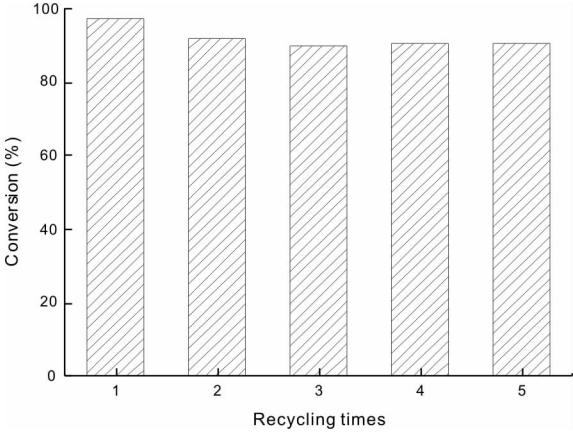
图 7 催化剂的重复使用性
