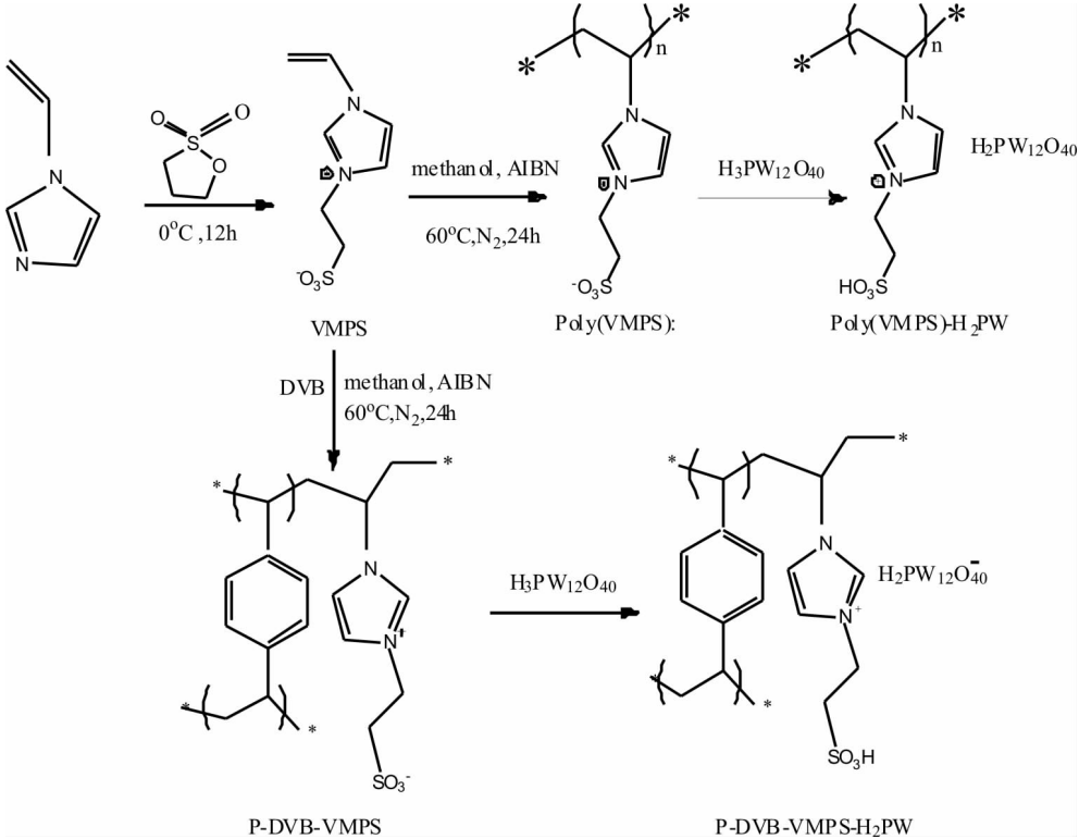
图1 催化剂合成示意图
