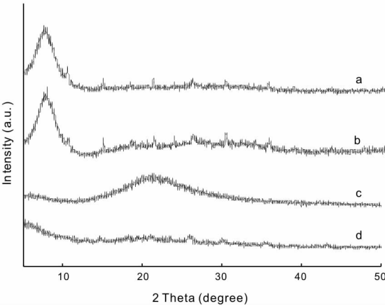
图3 不同杂多化合物催化剂的XRD谱图 (a) Poly(VPIM)-H 2 PW; (b) Poly(VMCA)-H 2 PW; (c) Poly(VMPS); (d) Poly(VMPS)-H 2 PW
